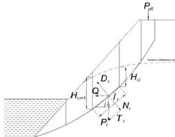
Рисунок 2. Расчет устойчивости обводненного изотропного откоса с учетом воздействия сейсмических сил методом алгебраического сложения сил
