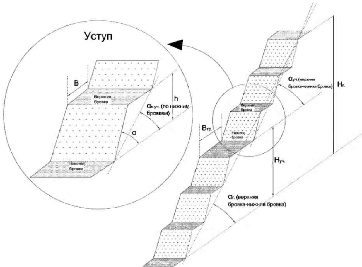
Рисунок 1. Схема конструкции бортов и уступов: h , H_{уч} , H_{г} – соответственно высота уступа, групп уступов, борта; \alpha , \alpha_{уч} , \alpha_{к.уч} , \alpha_{г} – соответственно, угол откоса уступа, угол откоса группы уступов, конструктивный угол откоса группы уступов и угол откоса борта карьера, разреза; B , B_{тр} – соответственно, ширина предохранительной и транспортной бермы
