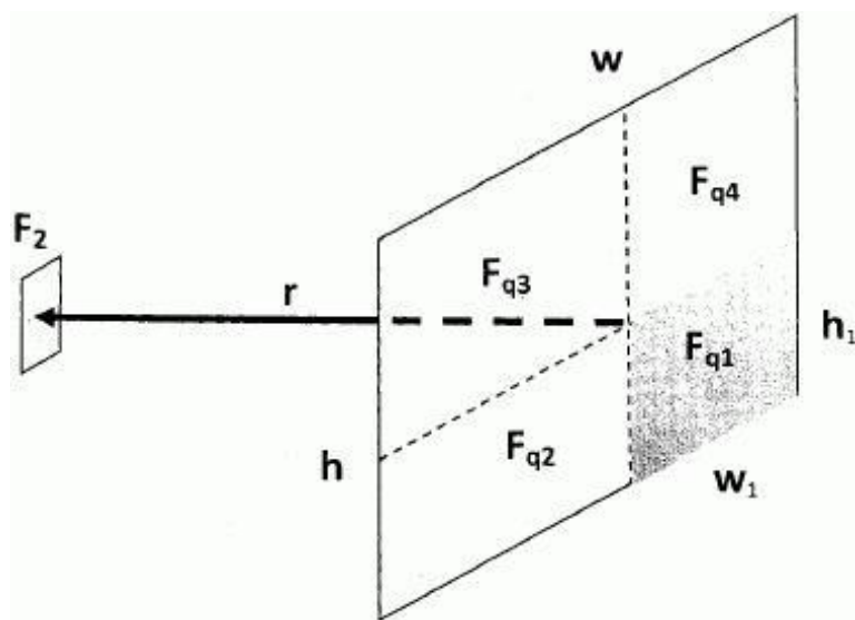
Рисунок А.3.2. Расположение излучающих поверхностей пламени Fq1-q4 и облучаемой поверхности материала соседнего объекта F2, где w1 и h1 - длина и ширина соответствующей части поверхности пламени.
